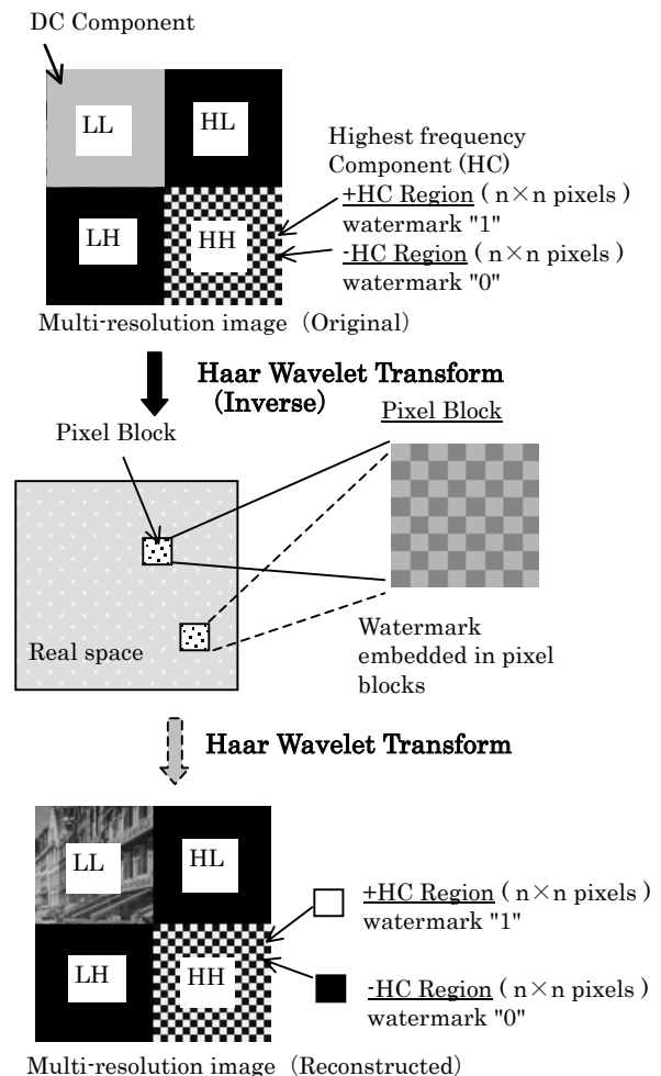
図1 光透かしの処理手順
