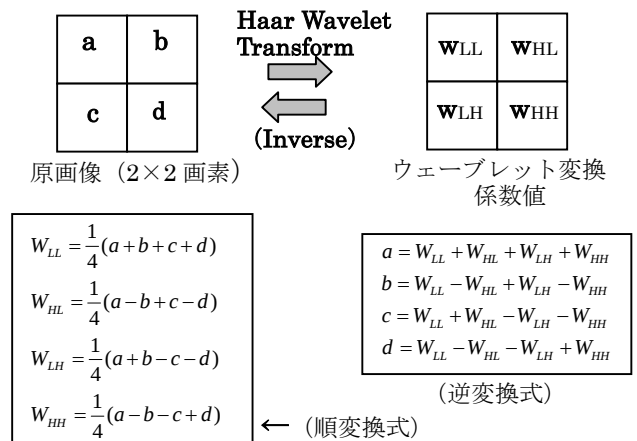
図2 2次元ハールウェーブレット変換
